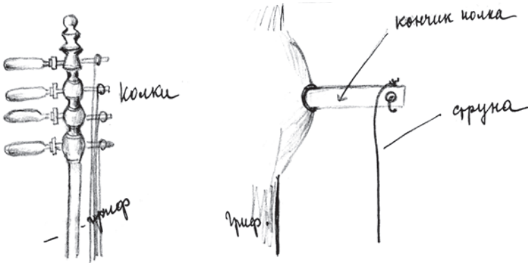
Рис. 68. Схема крепления струн на «пызанчи» [рисунок из рукописи Е.Д. Прокофьевой]
