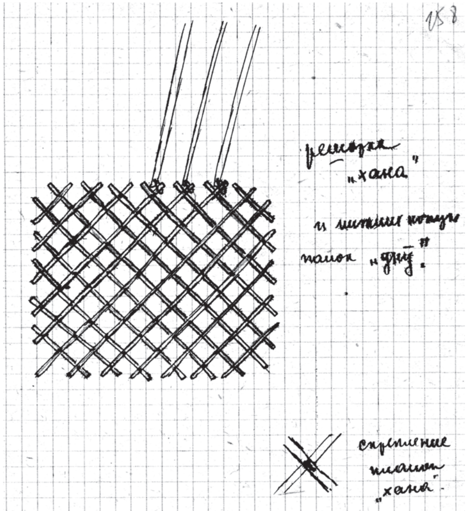
Рис. 26. Схема крепления «стенок»-решеток юрты [рисунок из рукописи Е.Д. Прокофьевой]
