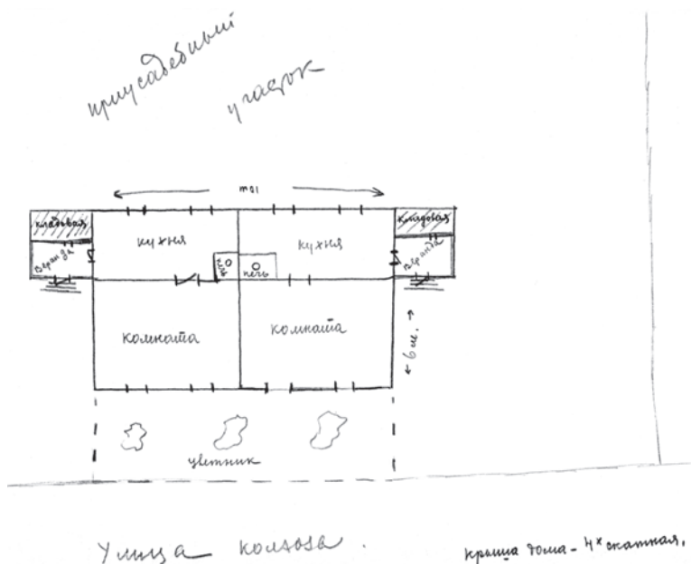
Рис. 35. Схема двухквартирного типового дома [рисунок из рукописи Е.Д. Прокофьевой]
