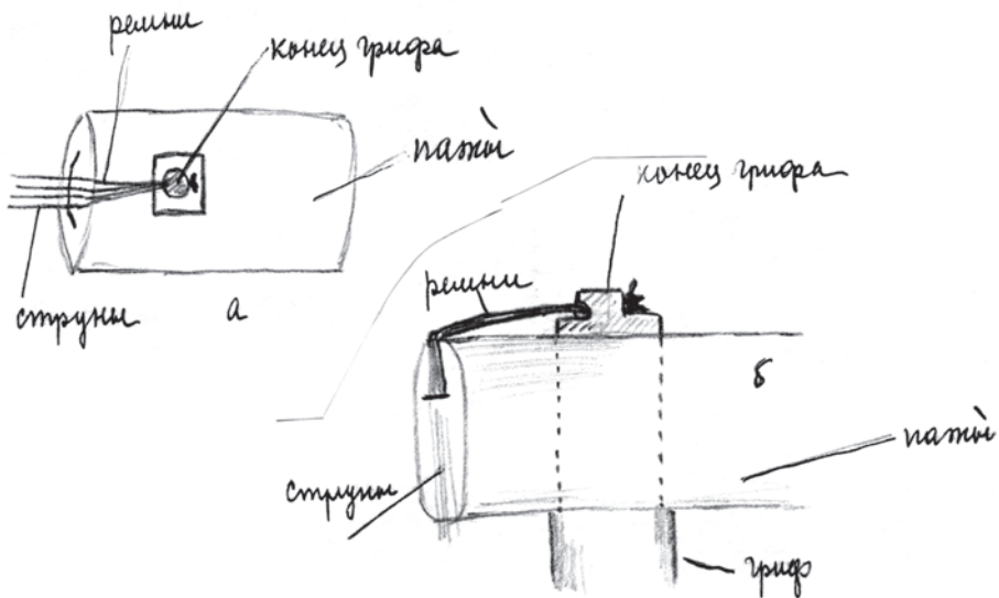
Рис. 67. Схема крепления струн на «пызанчи» [рисунок из рукописи Е.Д. Прокофьевой]
