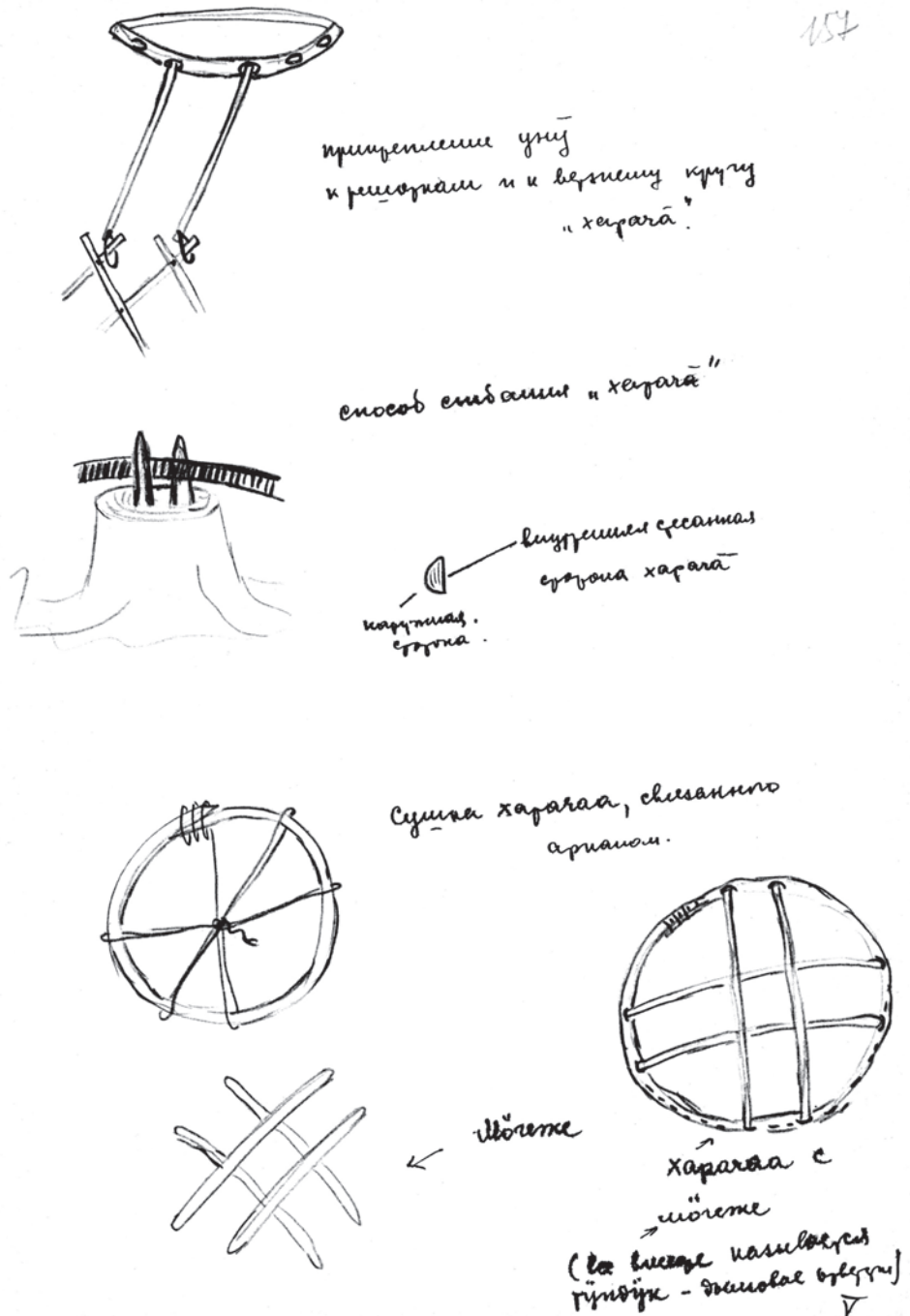
Рис. 27. Схема сборки верхней части каркаса юрты [рисунок из рукописи Е.Д. Прокофьевой]
