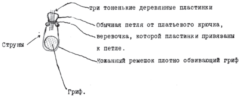
Рис. 69. Схема крепления струн на «пызанчи» [рисунок из рукописи Е.Д. Прокофьевой]
